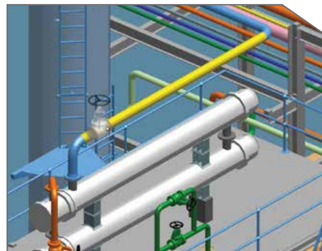
Thiết mềm AutoCad thiết kế gia công đường ống AutoCad software for pipeline design and processing 用于管道设计和处理的 AutoCad 软件
