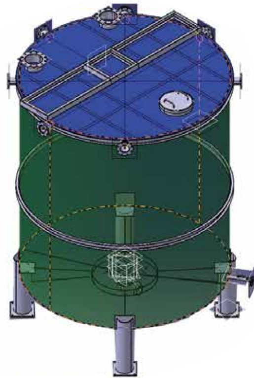
Thiết kế bồn inox bằng phần mềm Autonet Designing stainless steel tanks with Autonet software 使用 Autonet 软件设计不锈钢罐
